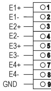
Analog Inputs
