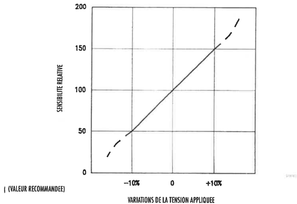
Fig. 3 - Rapport entre tension appliquée et sensibilité
