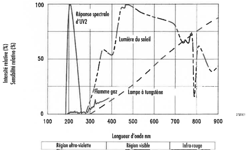
Fig. 2 - Sensibilité et background d'UV2
