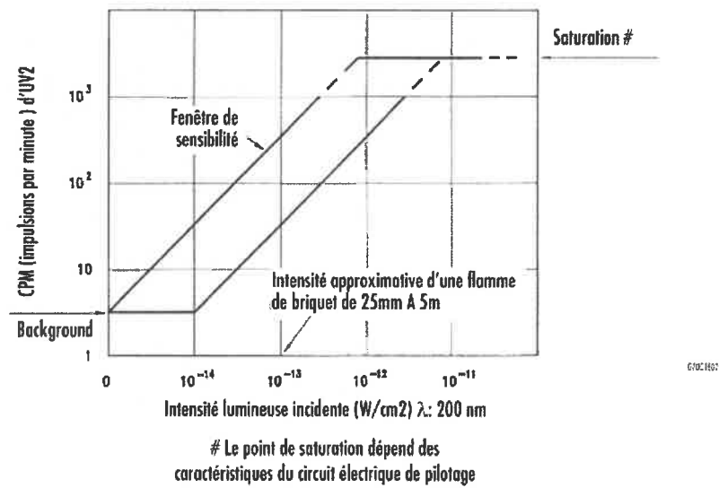
Fig. 2 - Sensibilité et background d'UV2
